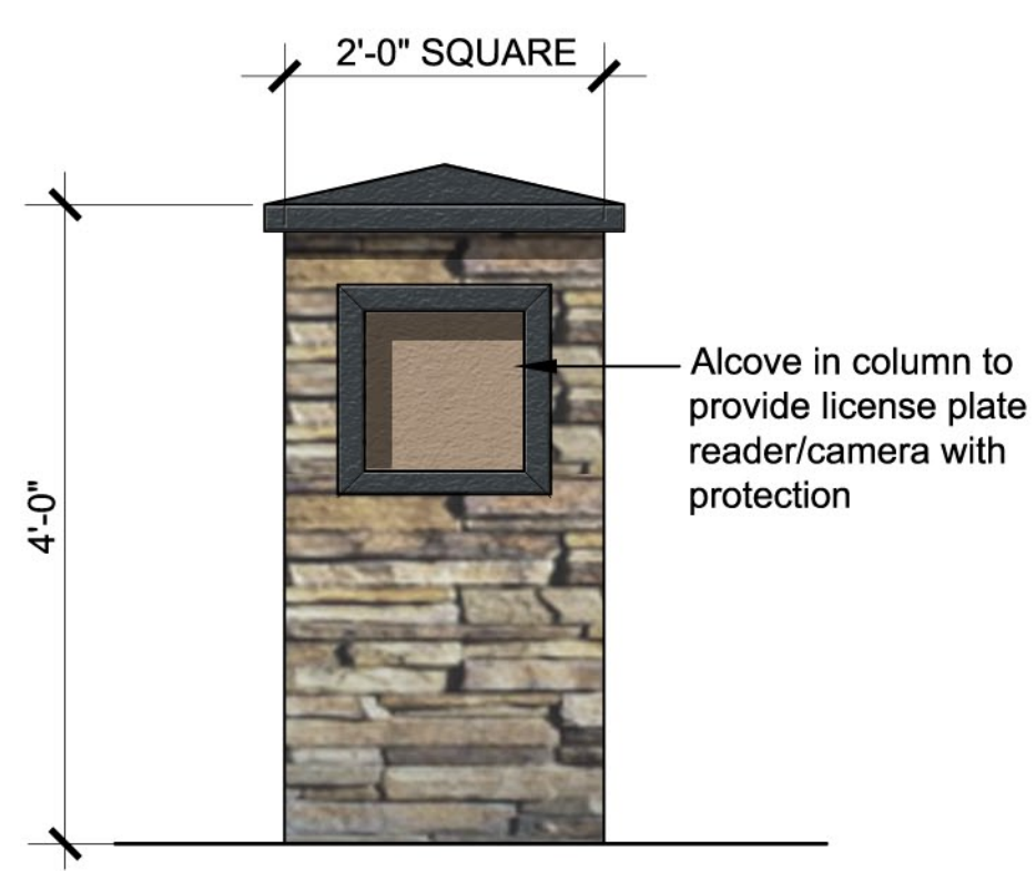
LPR COLUMN SCALE : 3/4"=1'-0"
